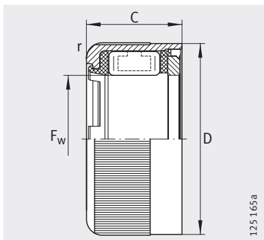
HFL0606-KF-R 3) , HFL0806-KF-R 3)
