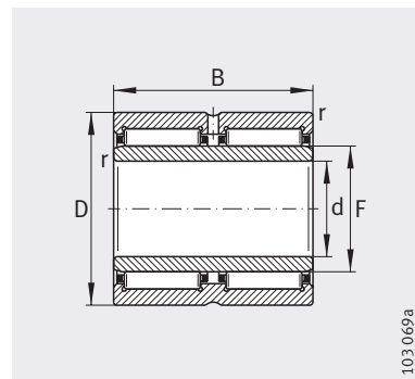
NA69...-ZW
