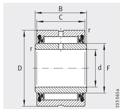
NA49..-2RSR
